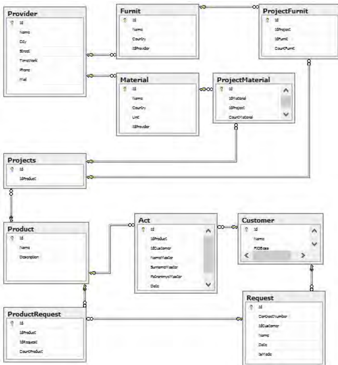
Рисунок 1 - Логическая модель БД системы ведения проектной деятельности ООО “Газпромнефть-Сахалин”
