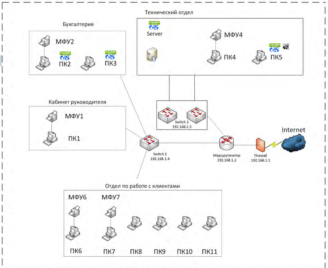
ITdiplom Рисунок 1 - Топология локальной сети ООО «Комлинк»
