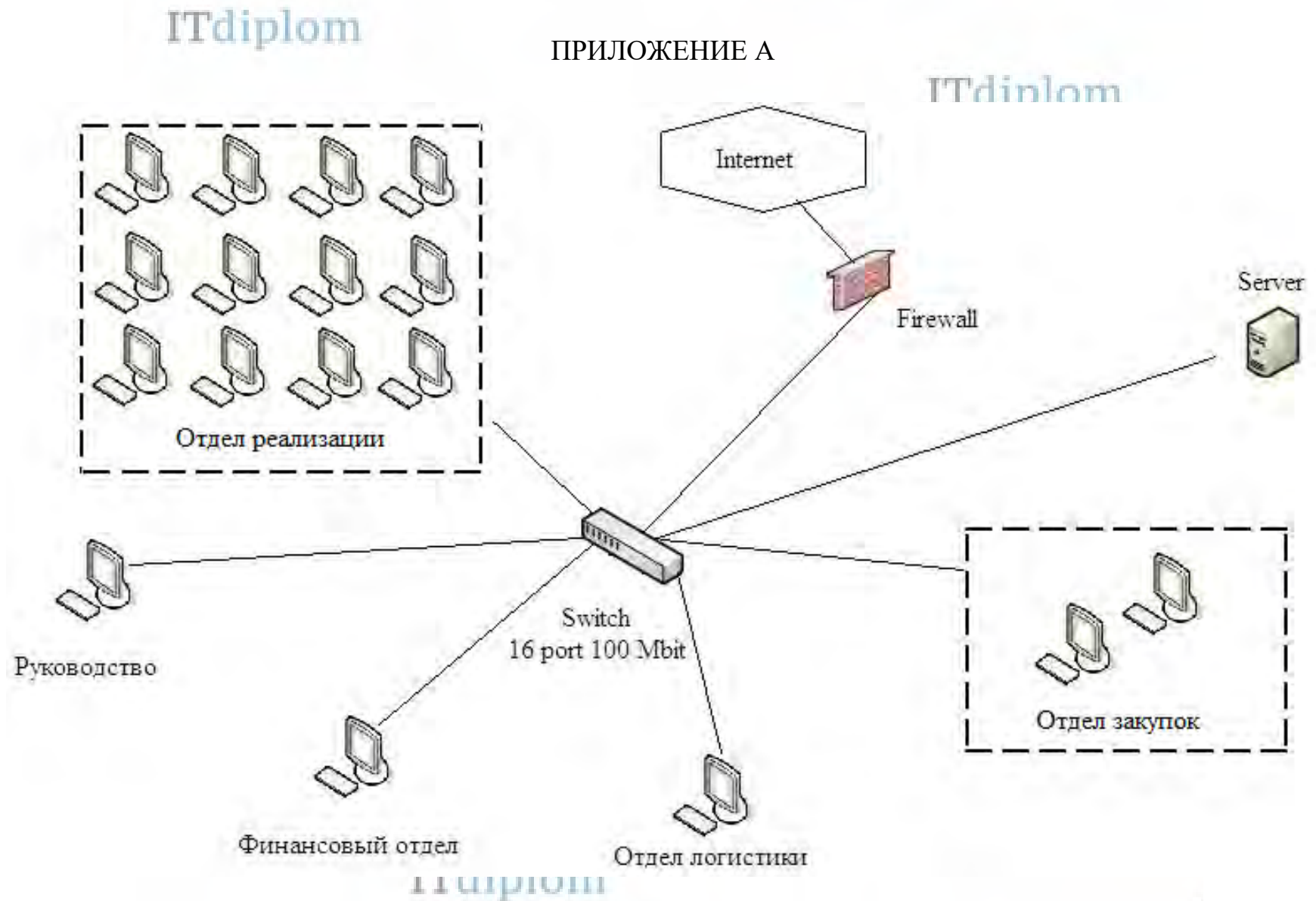
Рисунок 1 – Локальная вычислительная сеть ООО «Спецснаб-Юг»
